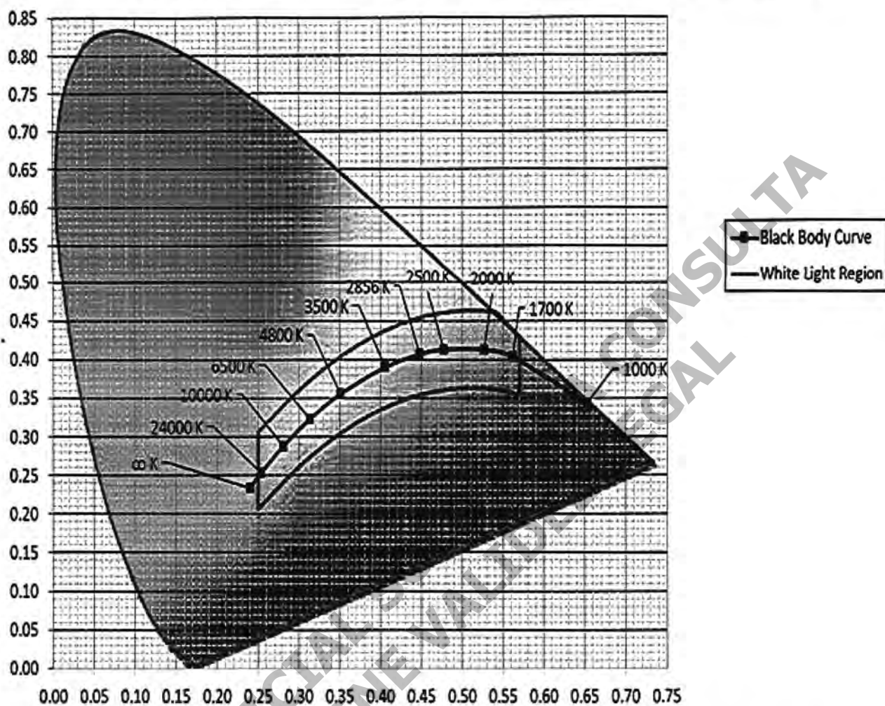
Figura 1: Diagrama de las ecuaciones de cromaticidad que definen la zona de emisión luminica, referencia CIE 1931.
