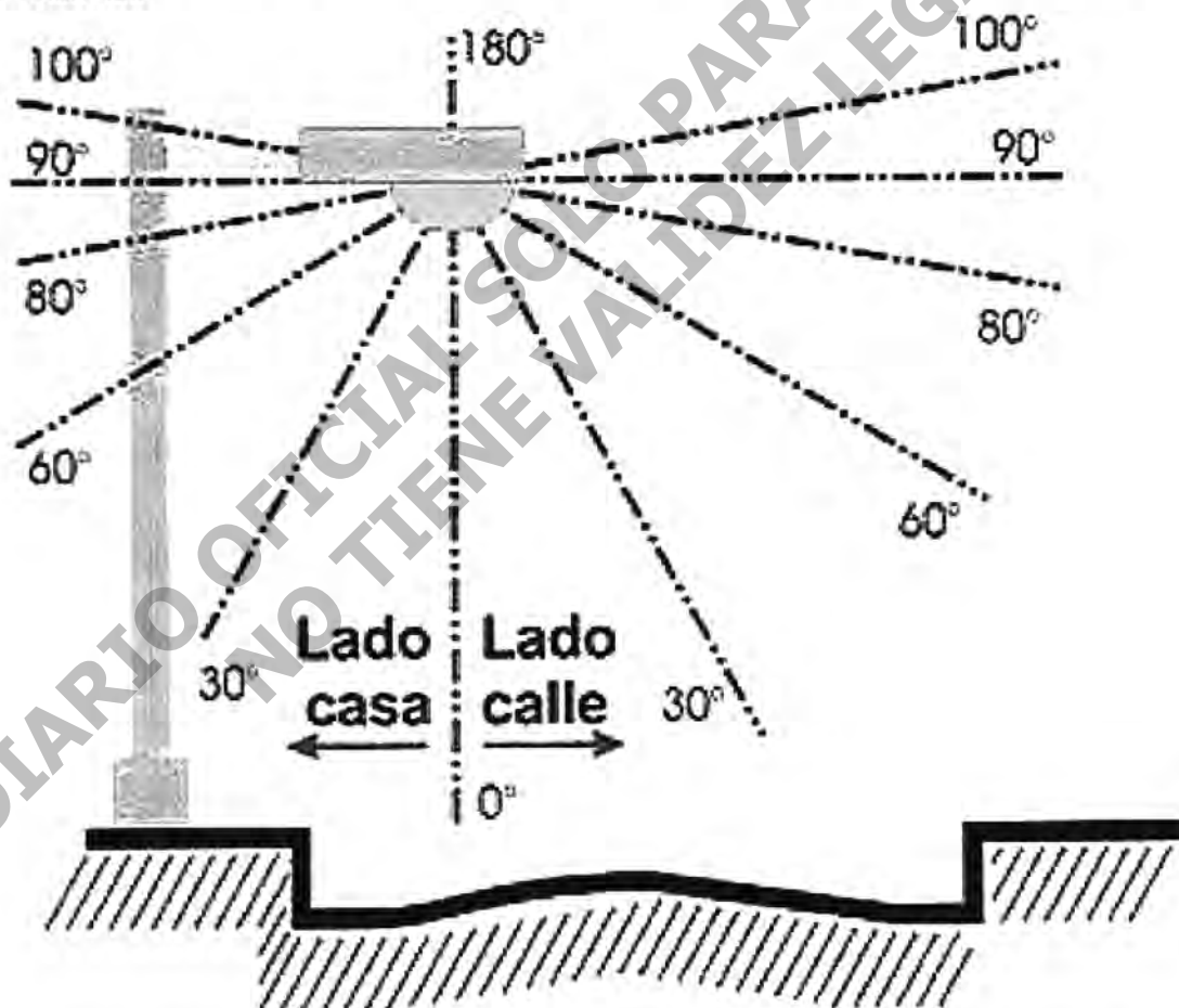
Figura 3. Ángulos de medición del flujo luminoso máximo, INTE E18-1:2020 Eficiencia Energética. Luminarias de diodos emisores de luz (LED) destinadas a alumbrado público. Parte 1: Requisitos
