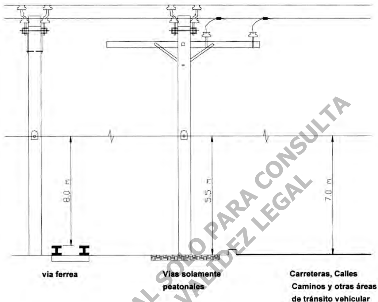
Figura No. 2 Libramientos mínimos para la instalación cables de telecomunicaciones.
