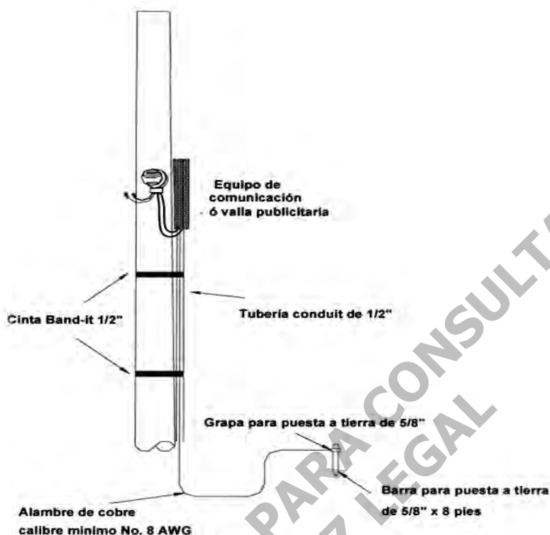
Figura No.4 Instalación de medidor en equipos en vallas publicitarias.
