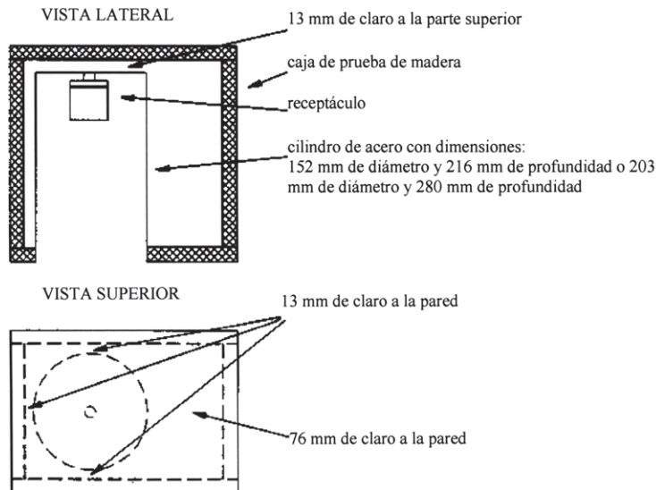
FIGURA A.1 Luminaria de prueba
